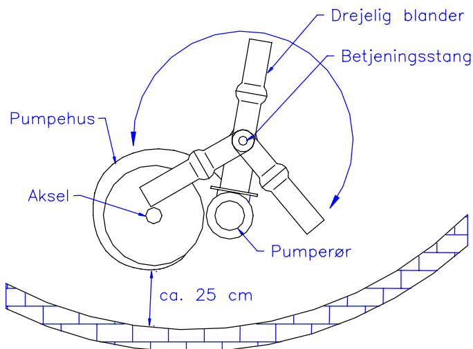
Fig.1 Pumpe med drejelig blander
