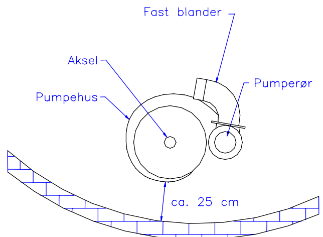
Fig.2 Pumpe med fast blander
