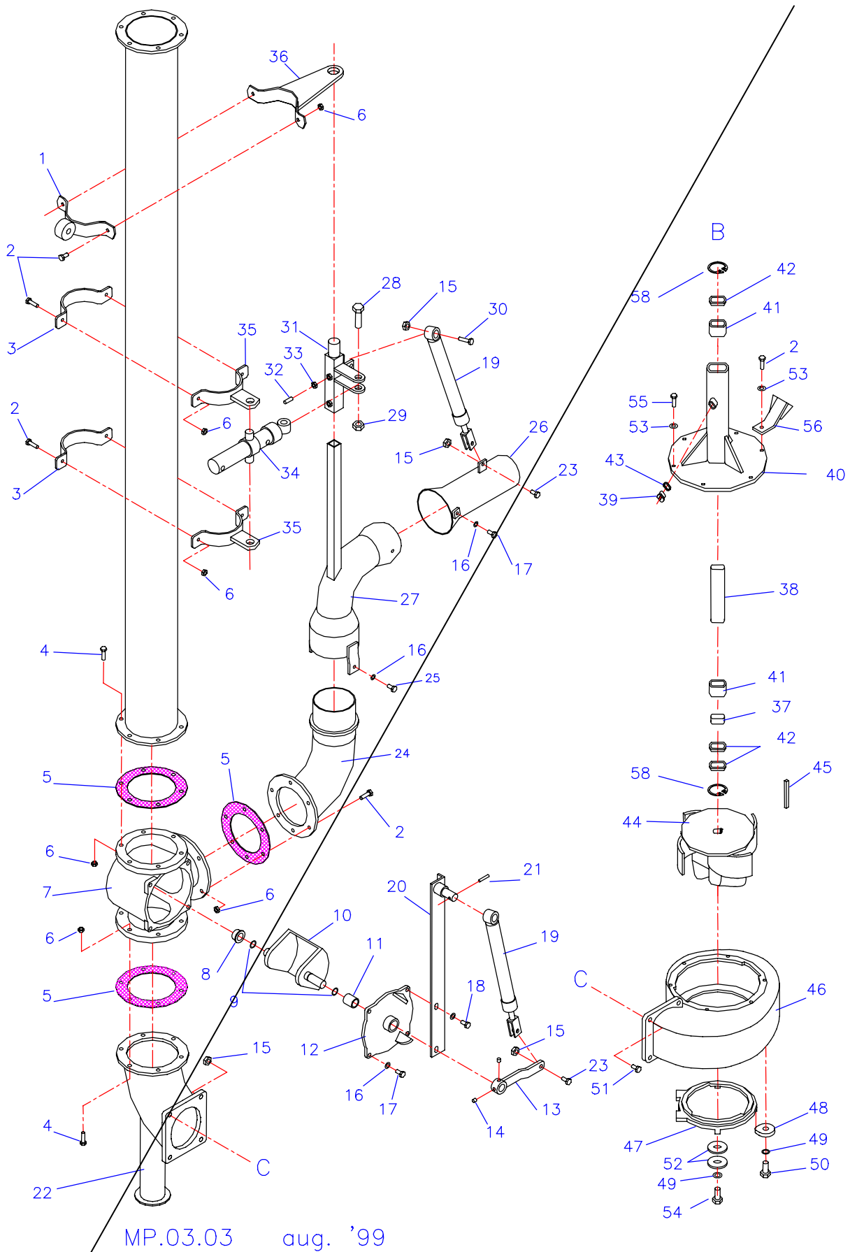
MULTIPUMPE - MP.03.03kh (KIMADANHANE fra jan. '04)
