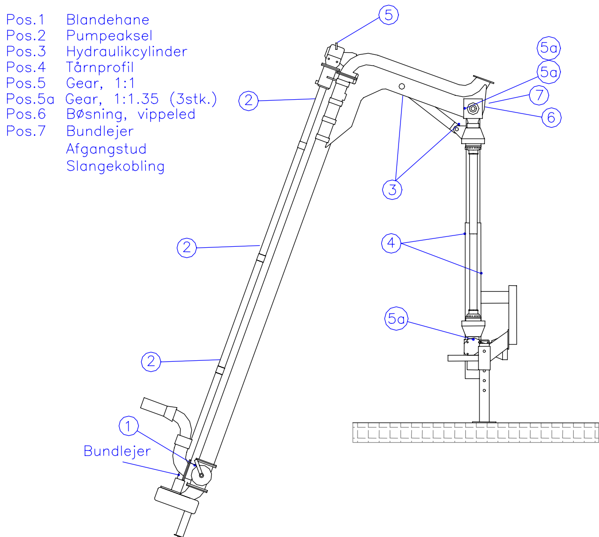
Figur 2: Smøresteder på Multipumpen
